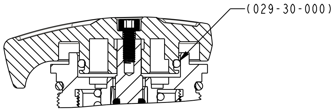
SECTION A-A SCALE 2.000
