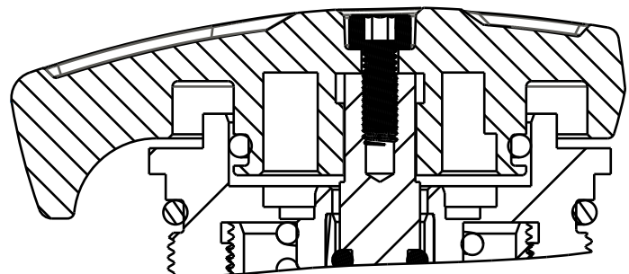
SECTION A-A SCALE 2.000
