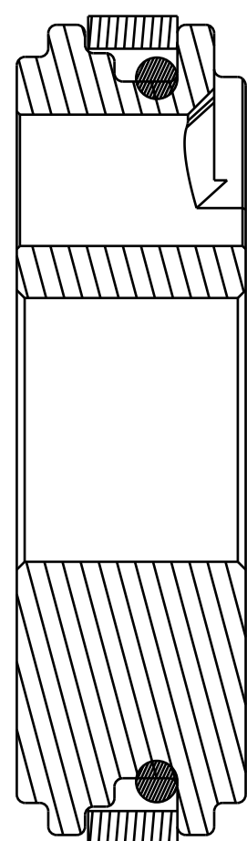
SECTION A-A
