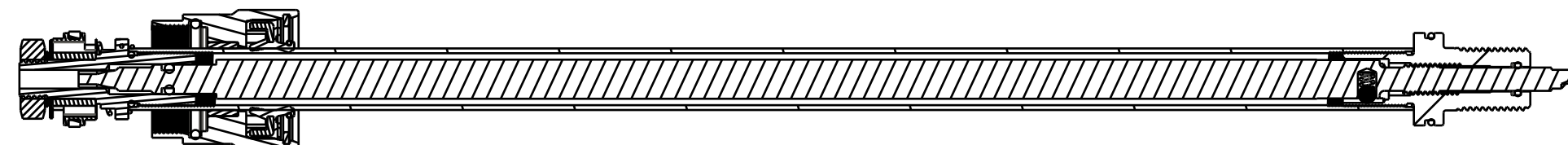
SECTION A-A
