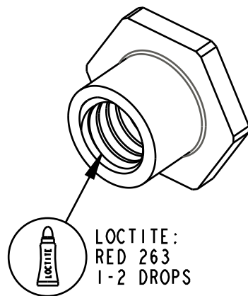
DETAIL Y
