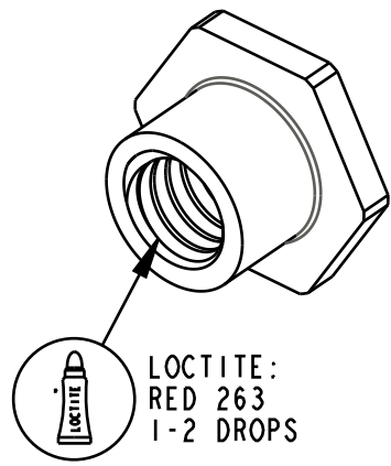
DETAIL Y SCALE 4:1
