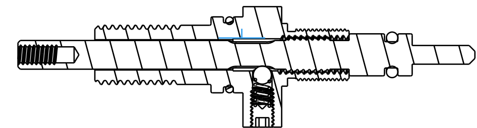
SECTION A-A SCALE 2.000
