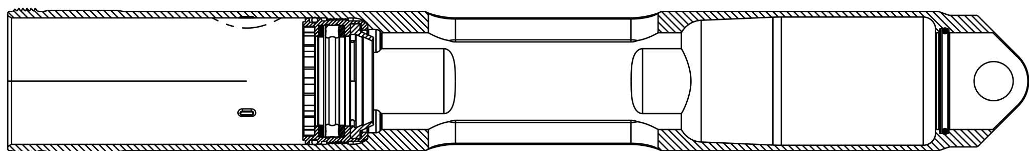
SECTION A-A
