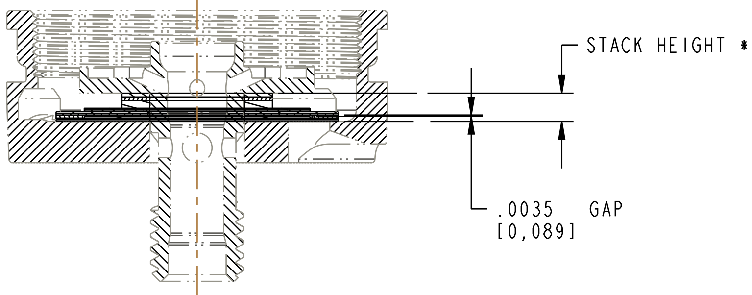
SECTION A-A SCALE 4:1
