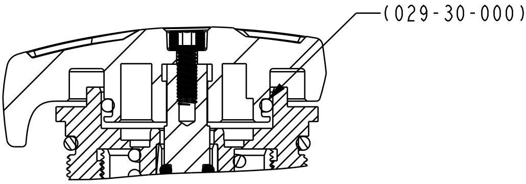
SECTION A-A SCALE 2.000
