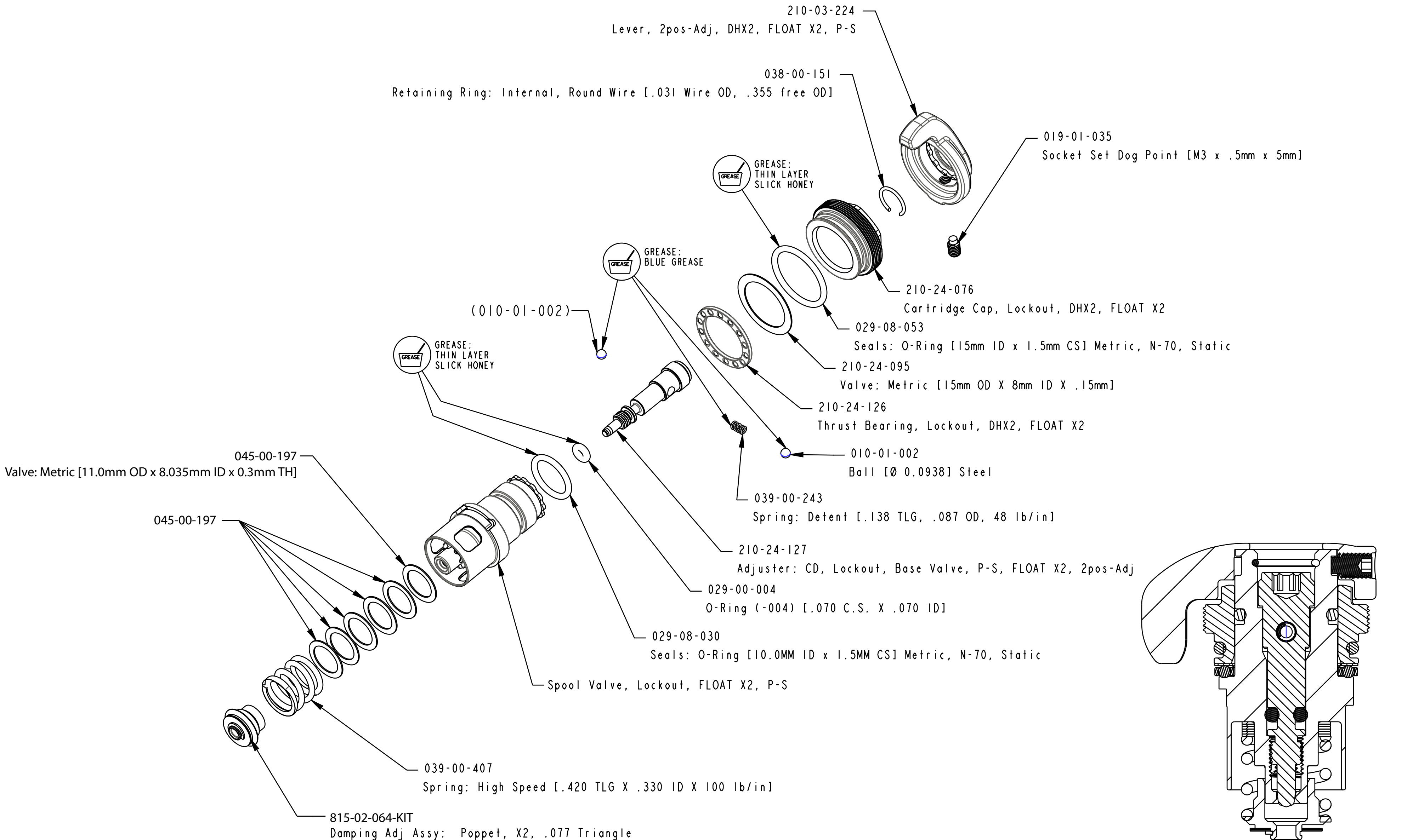
SECTION A-A SCALE 3.000
